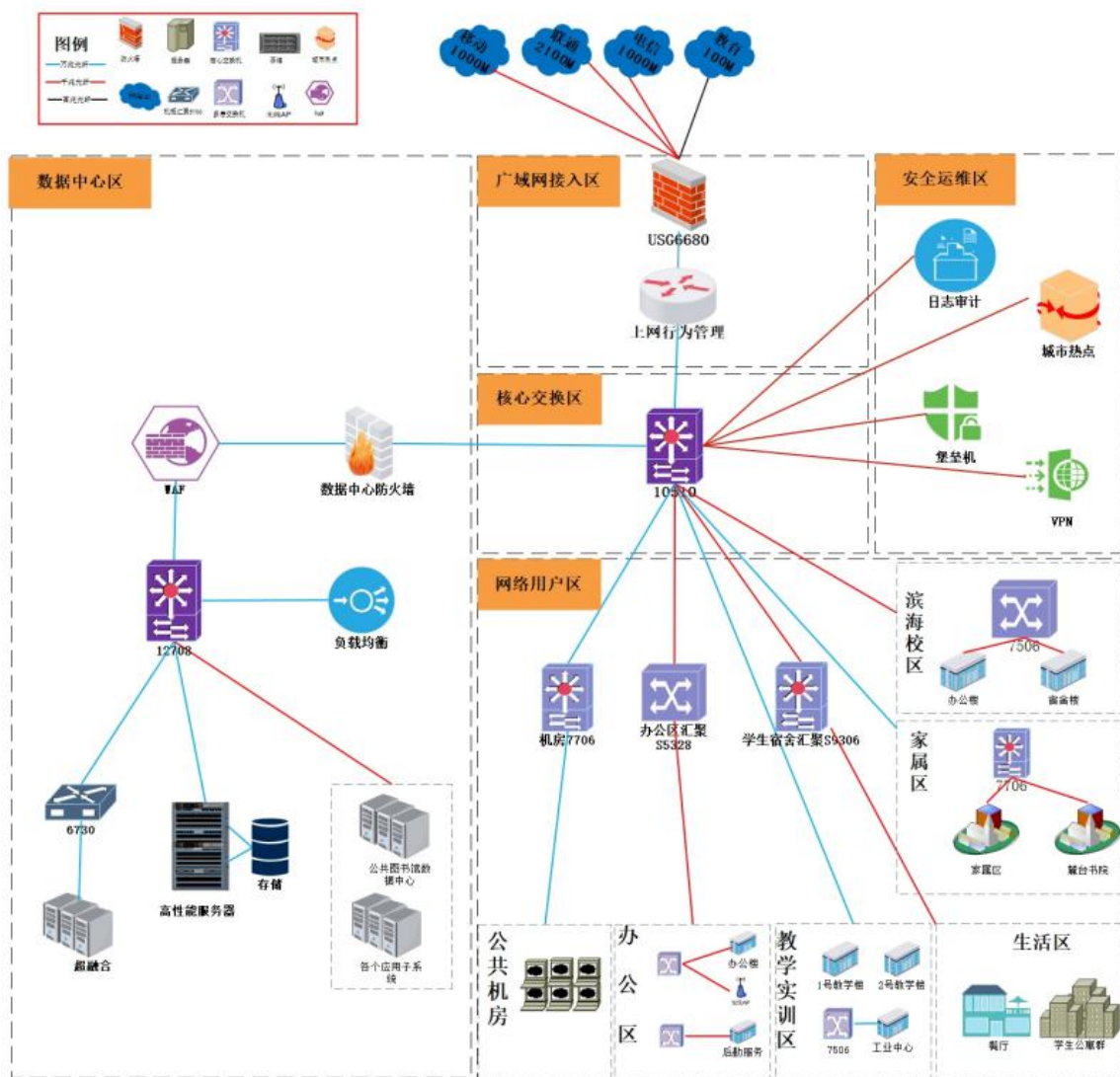
山东科技职业学院校园网络拓扑图
